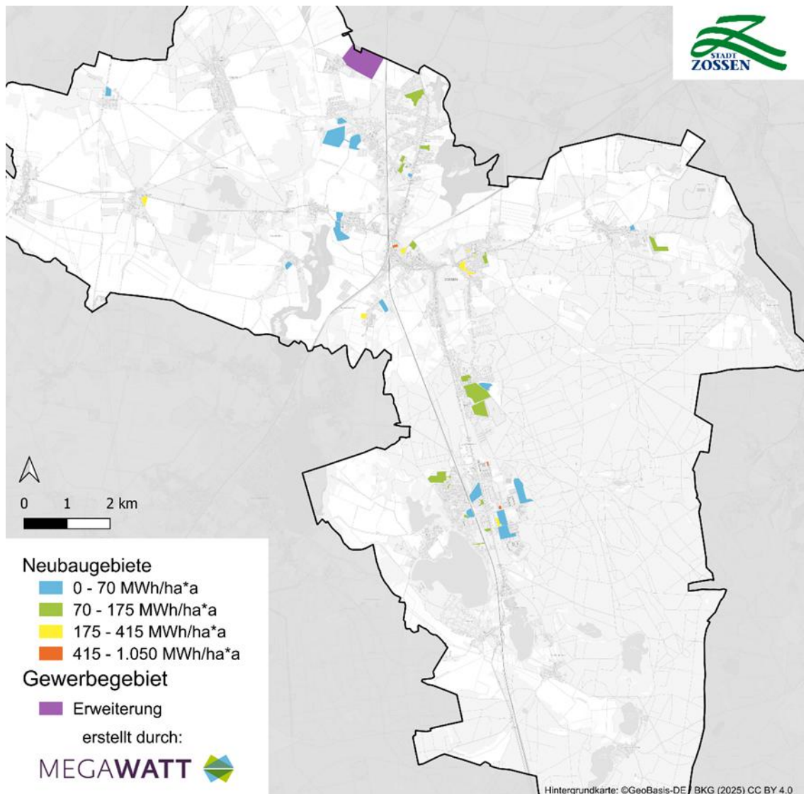
Abbildung 3: Geplante Neubauvorhaben im Stadtgebiet (ab einer Wärmedichte von 70 MWh/ha·a wird ein Wärmenetz bei Neubaugebieten empfohlen 2 )
